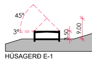
HÚSAGERÐ E-1
