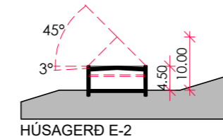
HÚSAGERÐ E-2
